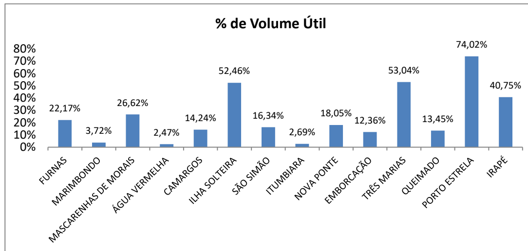
Figura 1 - Situação dos Reservatórios do Sistema Integrado Nacional – Dados de 19/11/2020
