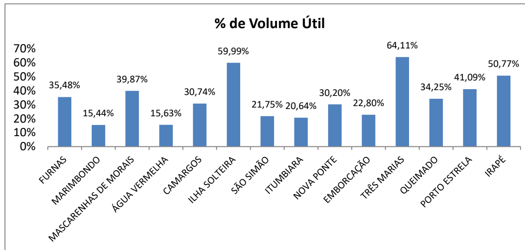
Figura 1 - Situação dos Reservatórios do Sistema Integrado Nacional – Dados de 08/10/2020
