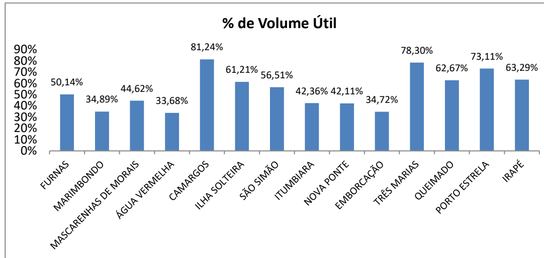
Figura 1 - Situação dos Reservatórios do Sistema Integrado Nacional – Dados de 27/08/2020
