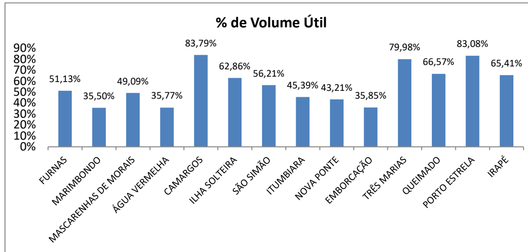
Figura 1 - Situação dos Reservatórios do Sistema Integrado Nacional – Dados de 20/08/2020
