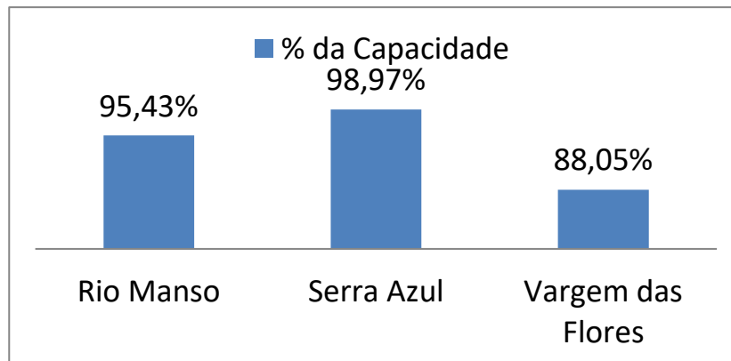
Figura 2 - Situação dos Reservatórios do Sistema Paraopeba – COPASA – Dados de 16/07/2020
