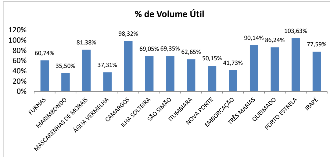
Figura 1 - Situação dos Reservatórios do Sistema Integrado Nacional – Dados de 09/07/2020
