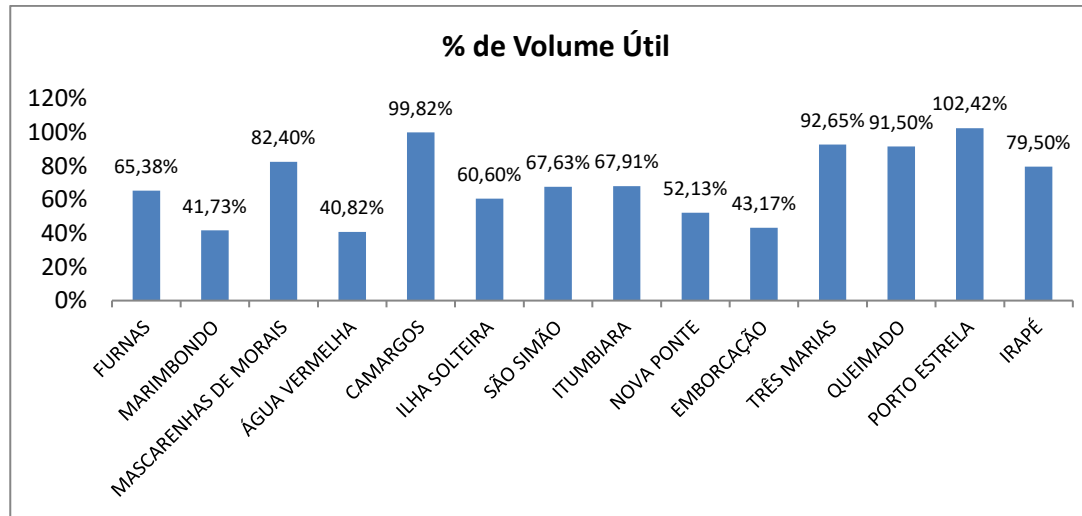
Figura 1 - Situação dos Reservatórios do Sistema Integrado Nacional – Dados de 25/06/2020
