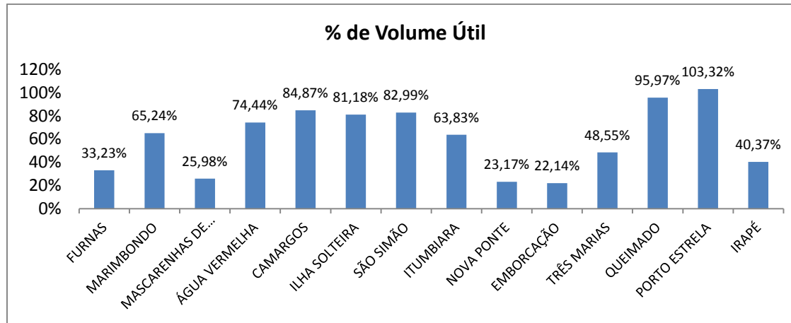
Figura 1 - Situação dos Reservatórios do Sistema Integrado Nacional – Dados de 10/05/2018
