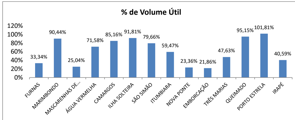
Figura 1 - Situação dos Reservatórios do Sistema Integrado Nacional – Dados de 19/04/2018
