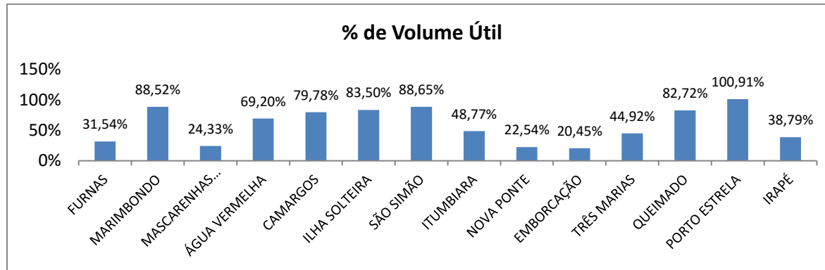
Figura 1 - Situação dos Reservatórios do Sistema Integrado Nacional – Dados de 27/03/2018
