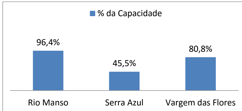
Figura 3 - Situação dos Reservatórios do Sistema Paraopeba – COPASA – Dados de 28/03/2018
