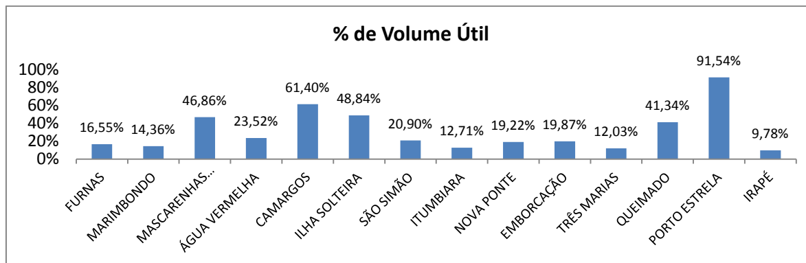
Figura 1 - Situação dos Reservatórios do Sistema Integrado Nacional – Dados de 10/10/2017
