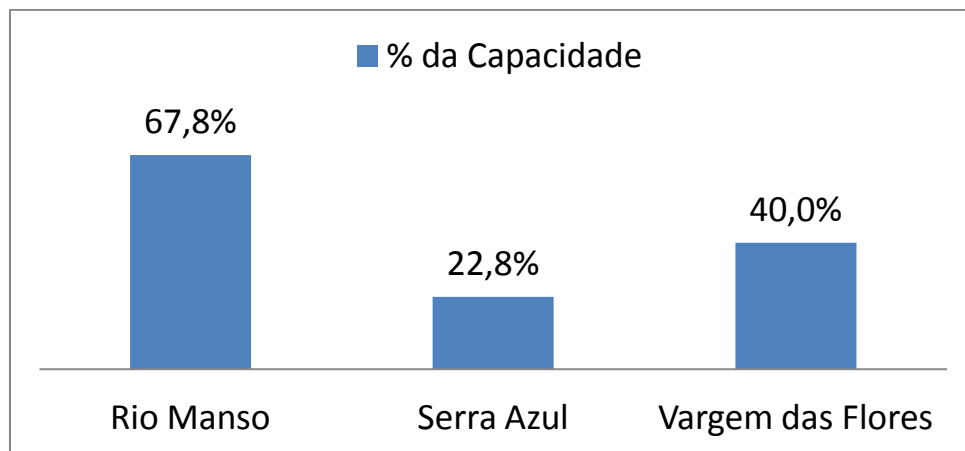
Figura 3 - Situação dos Reservatórios do Sistema Paraopeba – COPASA – Dados de 22/09/2017
