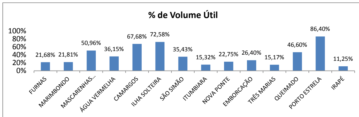
Figura 1 - Situação dos Reservatórios do Sistema Integrado Nacional – Dados de 21/09/2017
