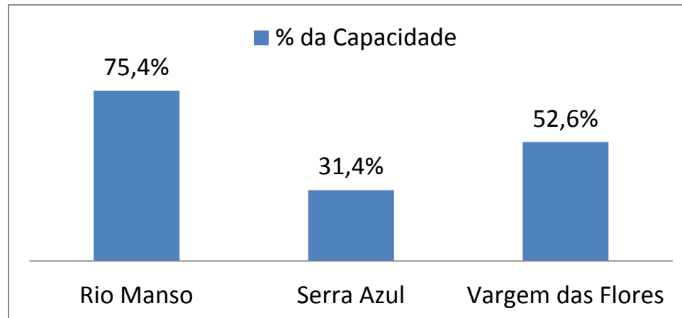
Figura 3 - Situação dos Reservatórios do Sistema Paraopeba – COPASA – Dados de 14/07/2017
