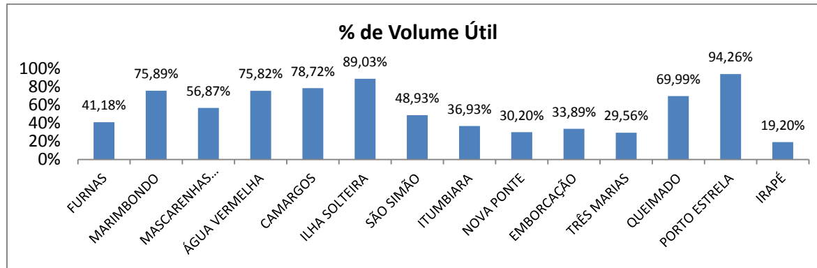
Figura 1 - Situação dos Reservatórios do Sistema Integrado Nacional – Dados de 09/06/2017
