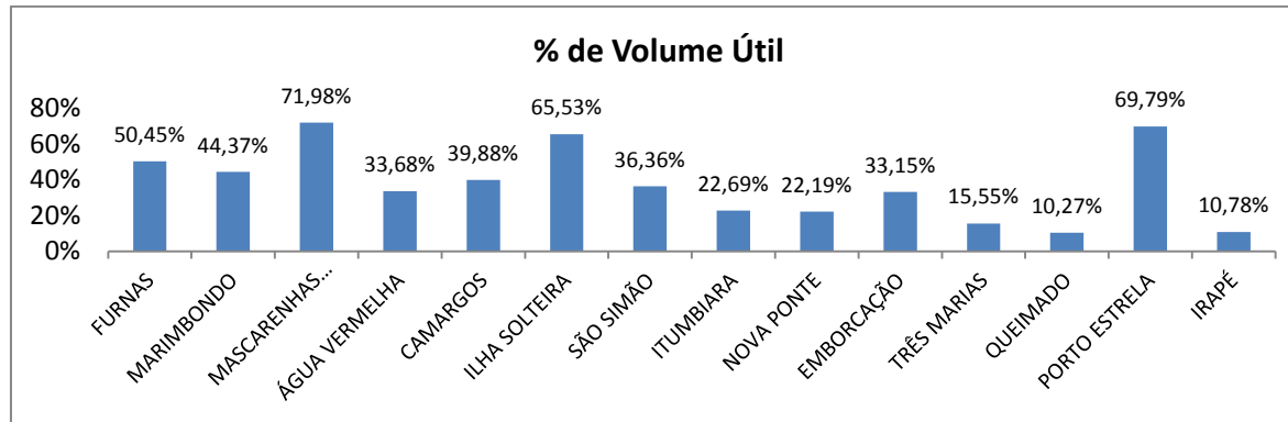
Figura 1 - Situação dos Reservatórios do Sistema Integrado Nacional – Dados de 24/11/2016
