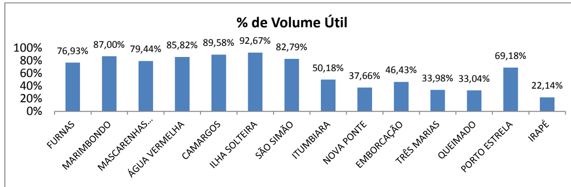
Figura 1 - Situação dos Reservatórios do Sistema Integrado Nacional – Dados de 14/07/2016
