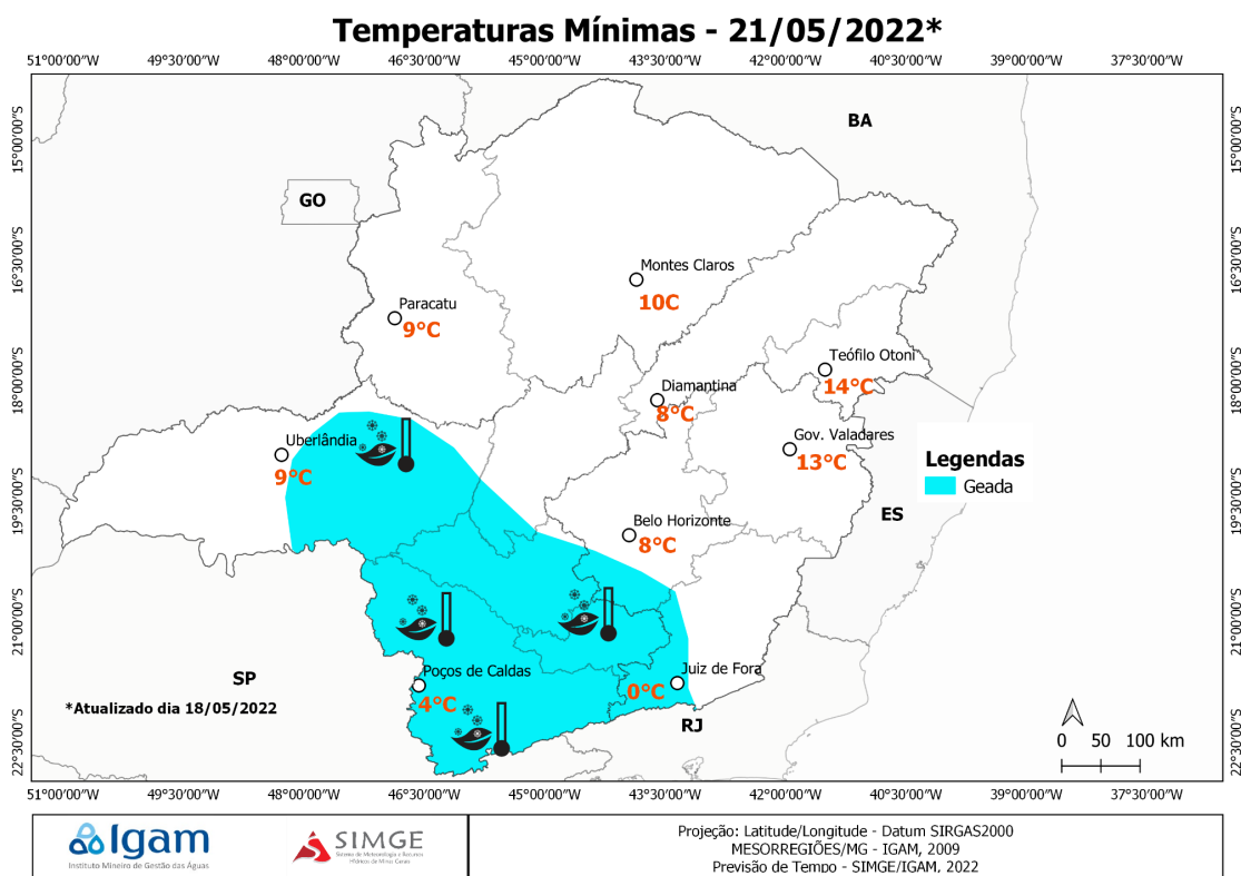
Figura 3: Mapa com as temperaturas mínimas previstas para a sexta-feira (21/05/2022), com destaque para as áreas com ocorrência de geada.
