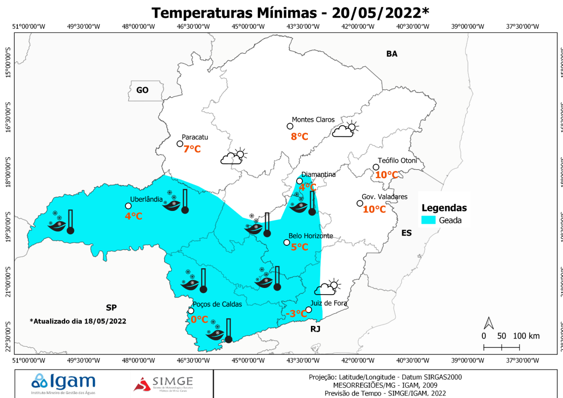
Figura 2: Mapa com as temperaturas mínimas previstas para a quinta-feira (20/05/2022), com destaque para as áreas com ocorrência de geada.
