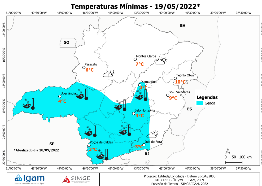
Figura 1: Mapa com as temperaturas mínimas previstas para a quarta-feira (19/05/2022), com destaque para as áreas com ocorrência de geada.
